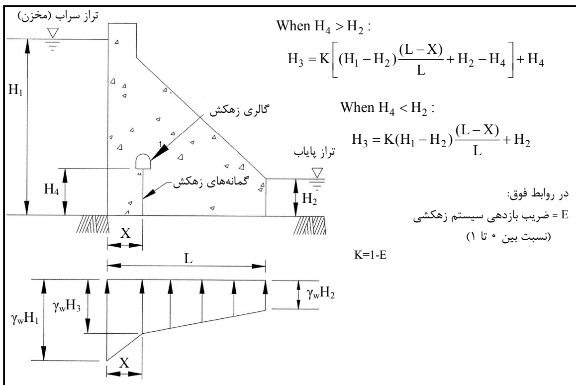
شکل ۷-۷- توزیع فشار برگشت در شرایط استفاده از پرده تزریق و سیستم زهکش
