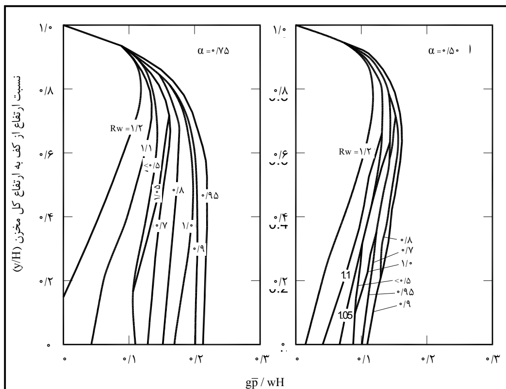
شکل ۸-۹- توزیع فشار هیدرو دینامیک (p(y)) در گام پنجم روش شبه دینامیکی چاپرا [۳۴]
