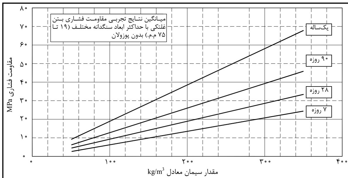
شکل ۳-۴- رابطه بین مقدار سیمان معادل و مقاومت فشاری- میانگین تجربیات موجود طرح‌های RCC بدون پوزولان [۱۹]
