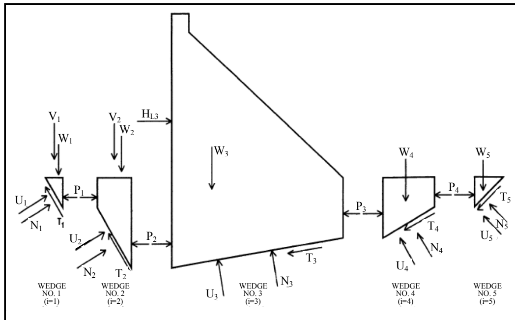
شکل ۷-۳- دیاگرام آزاد نیروهای وارد بر هر گوه در روش تحلیل لغزش چندگوهی [۲۷]
