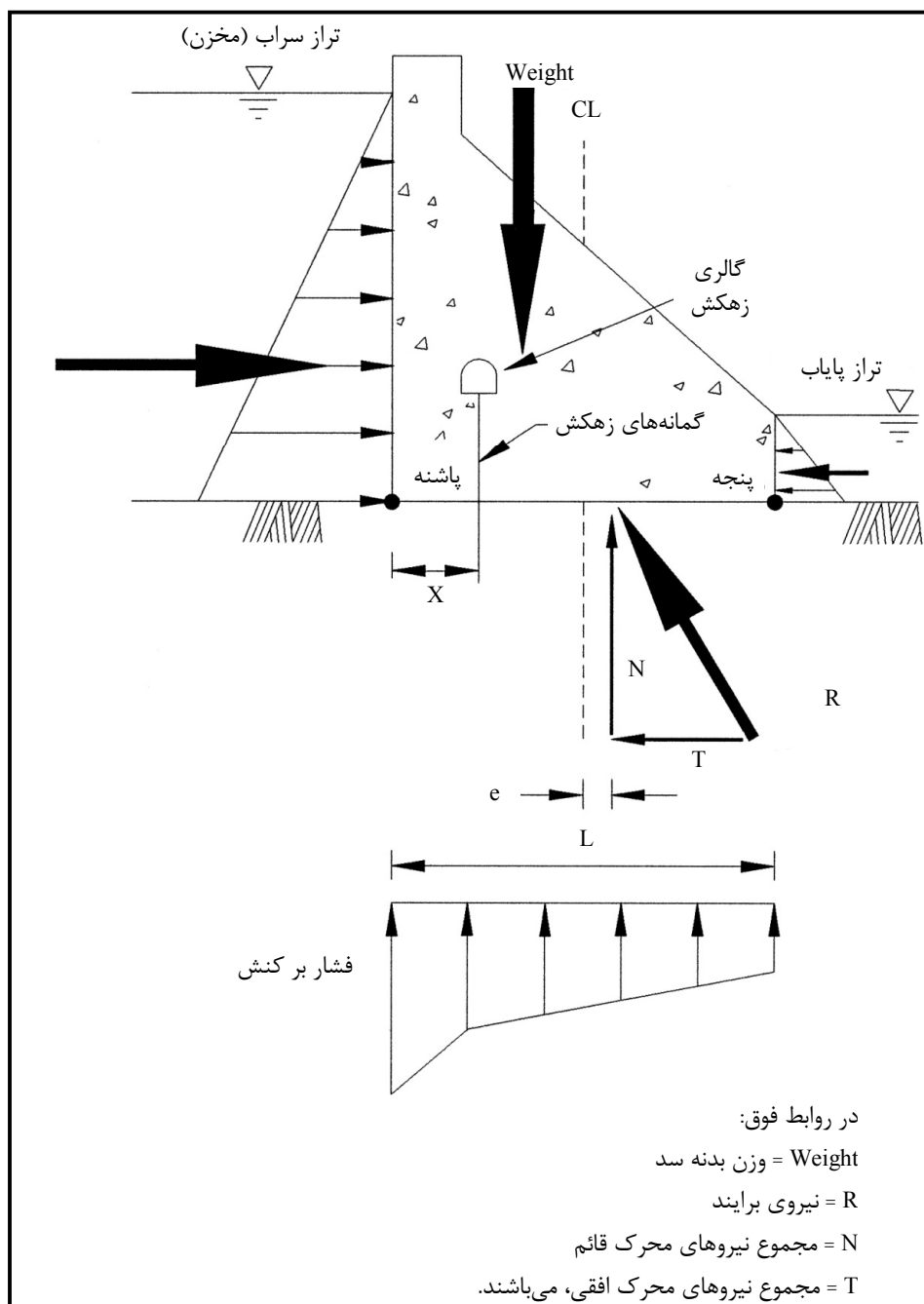
شکل ۷-۱- دیاگرام آزاد نیروهای وارد بر بدنه سد در روش تحلیل لغزش تک‌گانه‌ای [۲۷]
