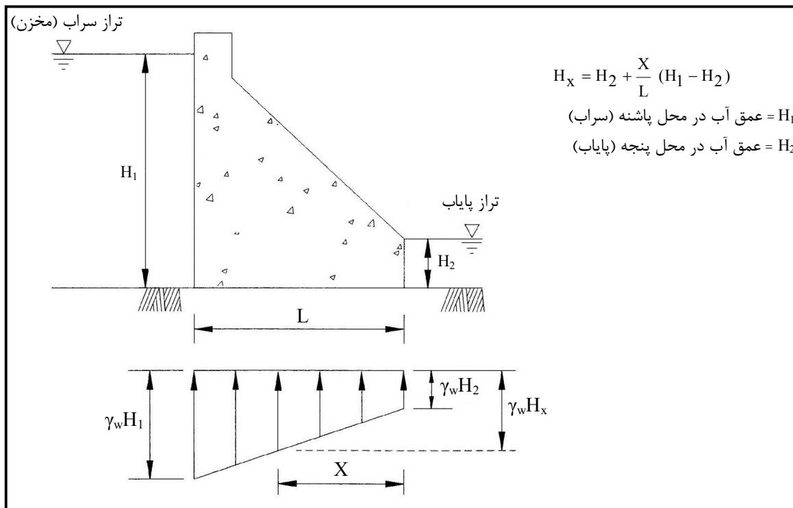
شکل ۶-۷- توزیع فشار برگشت در شرایط عدم وجود پرده تزریق و سیستم زهکش
