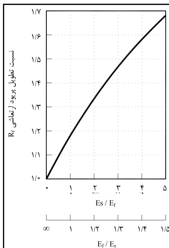
شکل ۹-۶- محاسبه نسبت پرود R_f در گام چهارم روش شبه دینامیکی چاپرا [۳۳]
