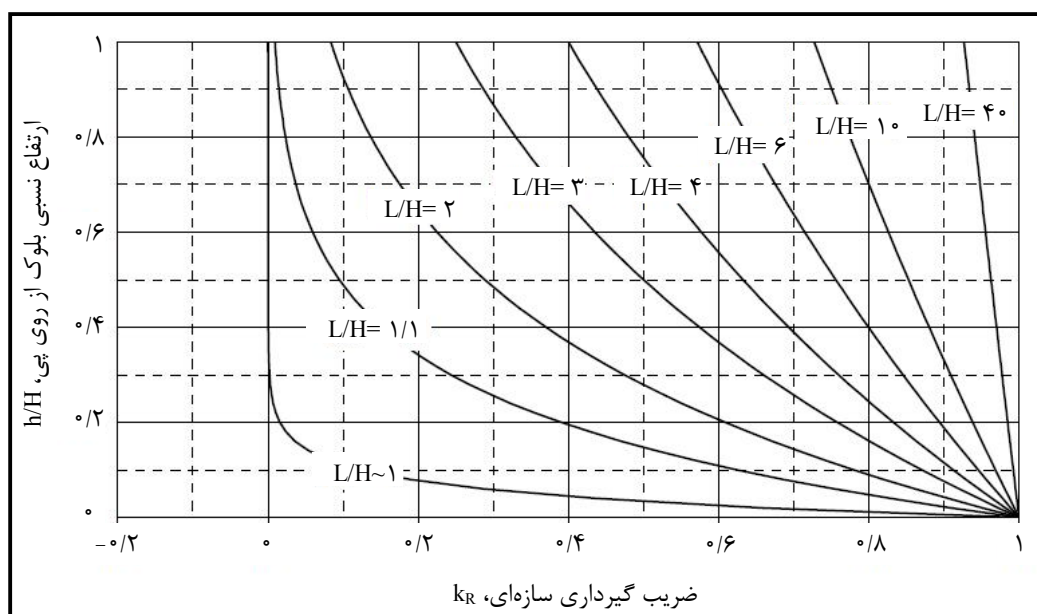
شکل ۸-۴- تغییرات ضریب گیرداری سازه‌ای بر اساس روابط پیشنهادی ACI- روابط ۸-۱۳ و ۸-۱۴
