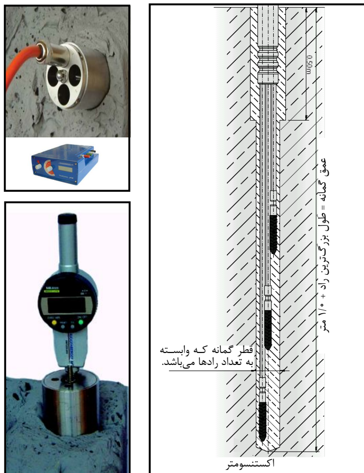
شکل ۱۰-۱- اکستنسومتر (سمت راست)، گنج قرائت اتوماتیک و گنج قرائت دستی آن [۱۱،۱۲]
