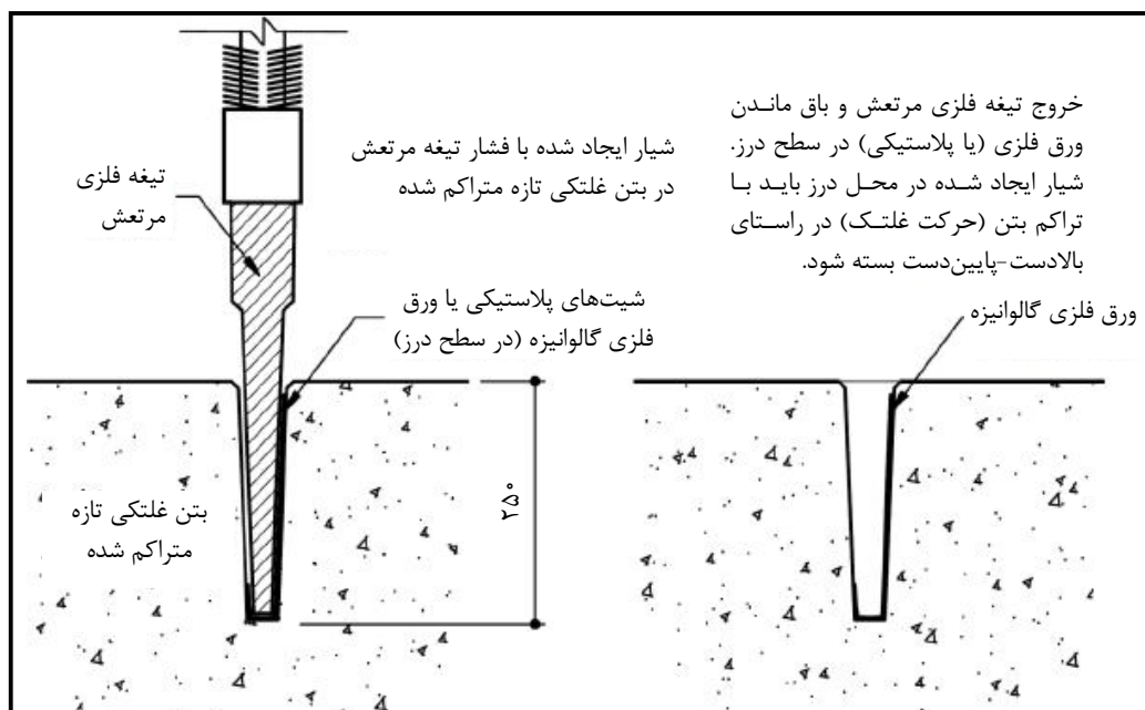
شکل ۵-۶- جزئیات روش اجرای درزهای انقباضی قائم در سدهای وزنی بتن غلتکی [۱۸]
