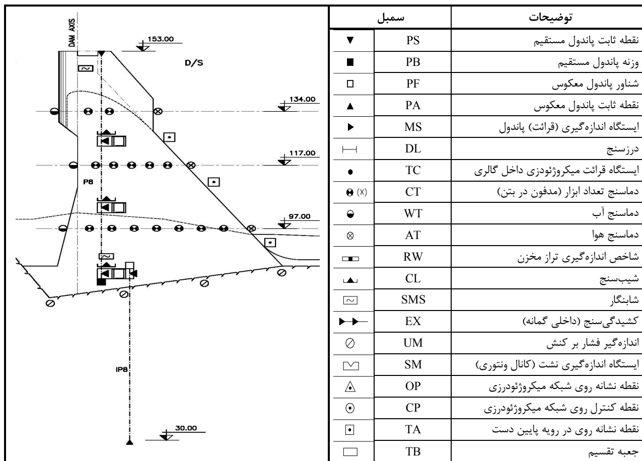
شکل ۱-۱۰ - سمت راست: لیست سمبل ابزارها، سمت چپ: شمای ابزار دقیق در مقطع طره مرکزی سد و پی (سد جگین) [۱۲]
