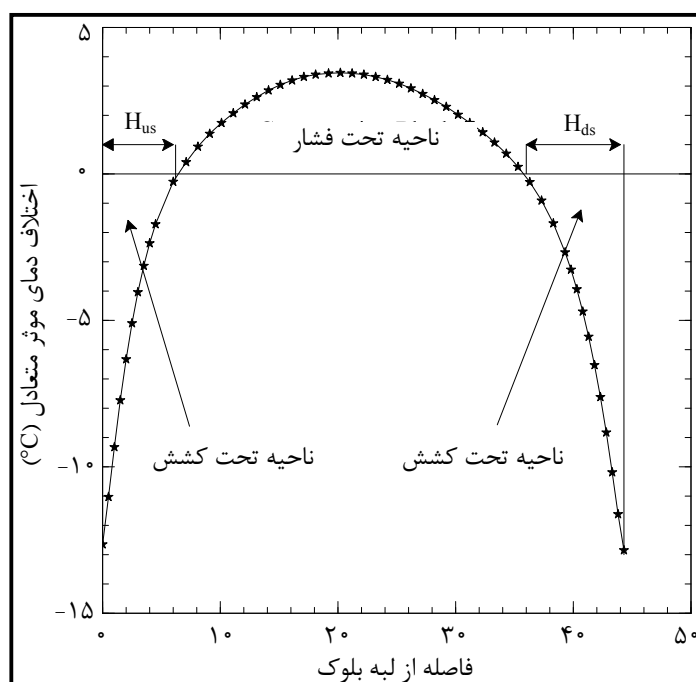
شکل ۸-۹- اختلاف دمای موثر (dT) در مقطع در زمان مورد نظر (سن ۳۶۵ روز)
