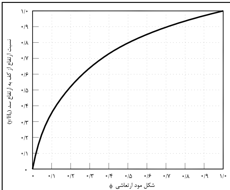
شکل ۷-۹- شکل مود اول (\phi(y)) در گام پنجم روش شبه دینامیکی چاپرا [۳۴]
