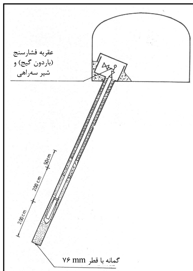
شکل ۱۰-۱۲- پیزومتر لوله بسته (Closed Standpipe Piezometers) برای اندازه‌گیری فشار برگشت [۱۱، ۱۲]
