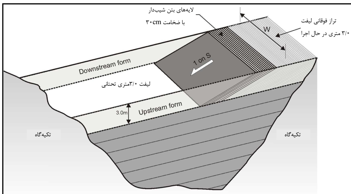
شکل ۵-۴- روش لایه شیب‌دار در سدهای بتن غلتکی (Sloped Layer Method - SLM) [۲۶]
