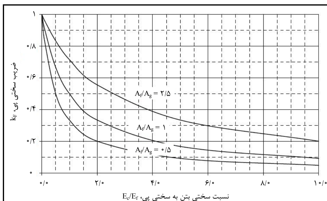
شکل ۸-۵- تغییرات ضریب گیرداری سازه‌ای بر اساس روابط پیشنهادی ACI- رابطه ۸-۱۵
