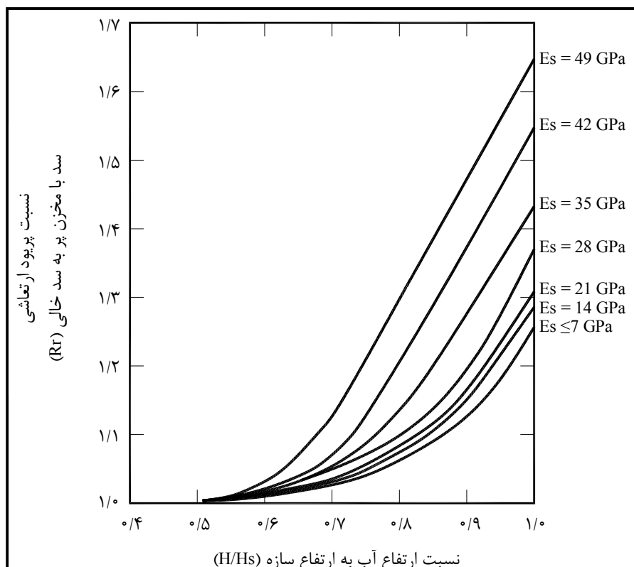
شکل ۹-۵- محاسبه نسبت پرود R_r در گام دوم روش شبه دینامیکی چاپرا [۳۴]
