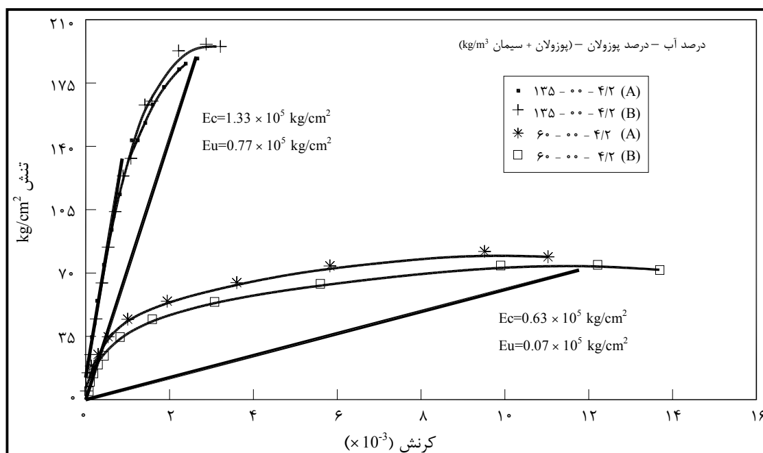
شکل ۸-۴ - مدول الاستیسیته وتری و مدول الاستیسیته نهایی بتن غلتکی [۱۸]
