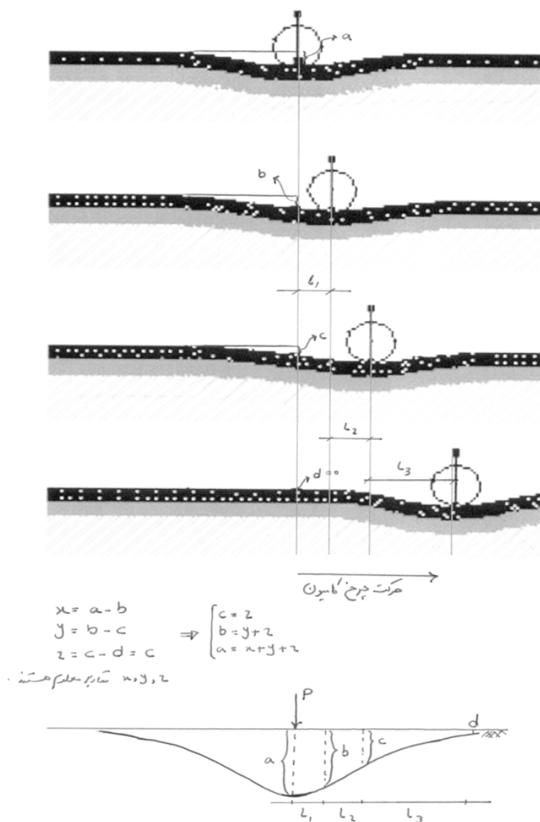
شکل ۵- ترسیم حوضچه تغییر شکل در آزمایش تیر بنکلمن
