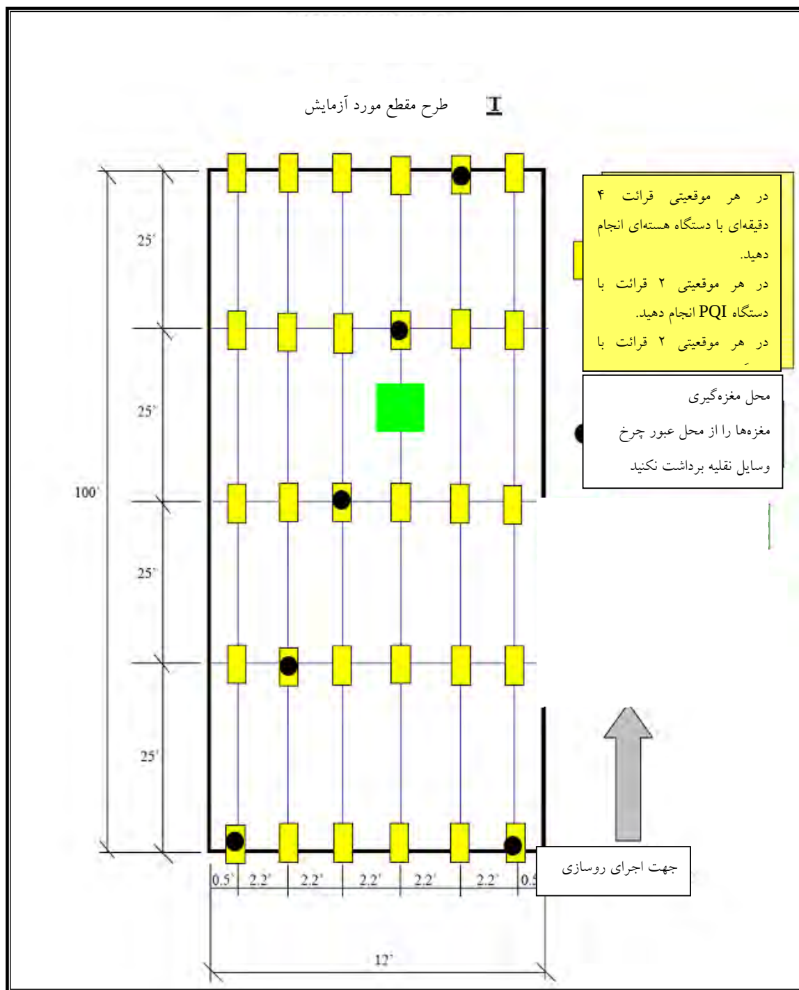
شکل ۸۴- موقعیت و نحوه آزمایش‌های انجام‌شده در هر قطعه آزمایش ۳۳ متری (۱۰۰ فوتی) و عرض ۳/۶۵ متری (۱۲ فوتی) [۶۹]
