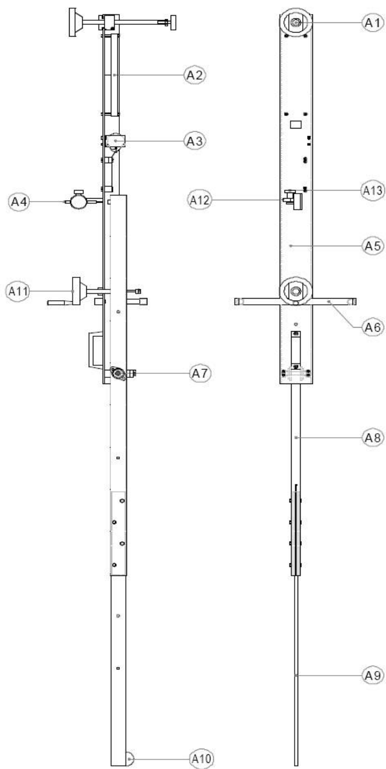
شکل ۴- جزییات بخش های تیر بنکلمن
