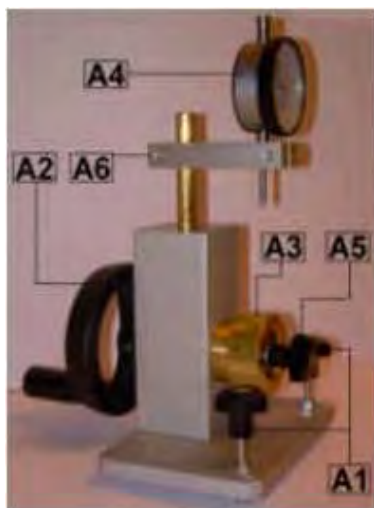
شکل ۷- تشریح جزییات دستگاه کالیبراسیون تیر بنکلمن
