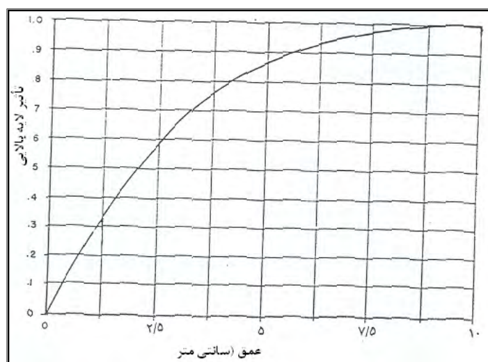
[۴۶] شکل ۴۶- تاثیر دانسیته سطحی در حالت پخش سطحی
