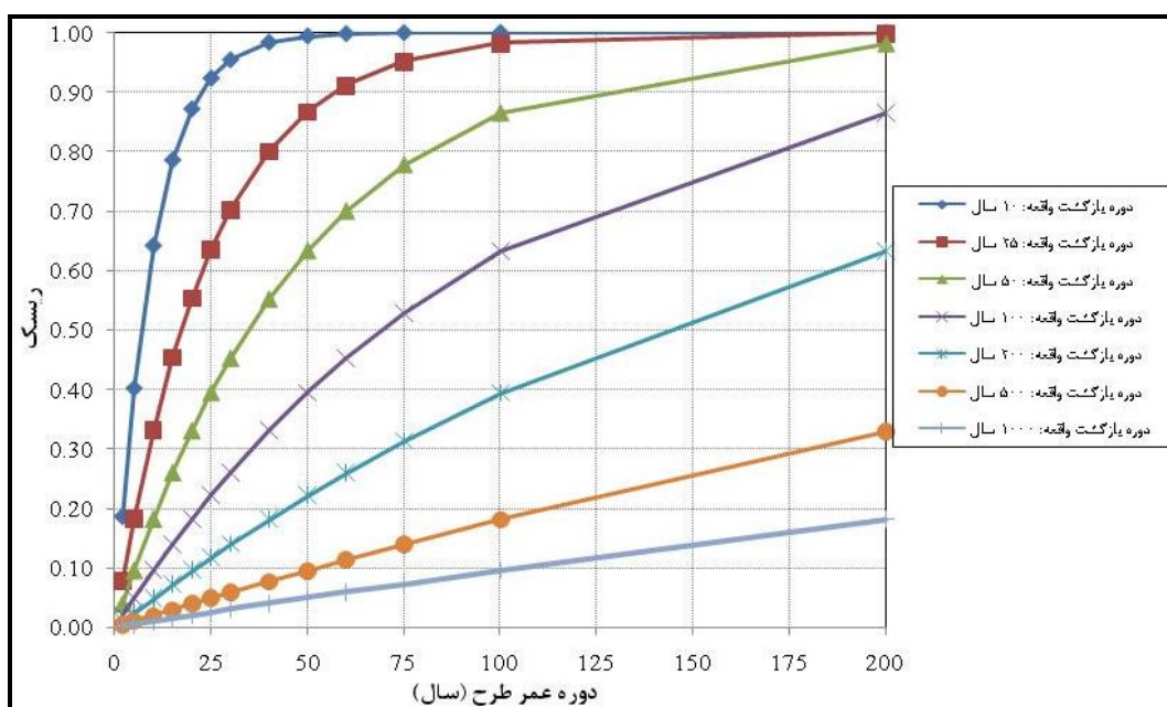
شکل ۱-۲- منحنی ریسک سیلاب برای دوره‌ی عمر مختلف طرح و دوره‌ی بازگشت مشخص- رخداد دوبار در سال
