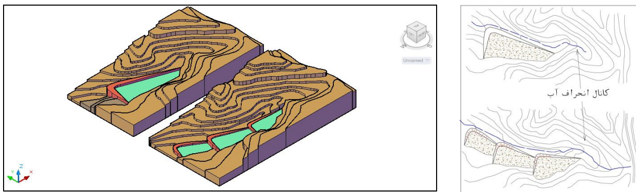
شکل ۳-۷- سدهای ته‌دره
