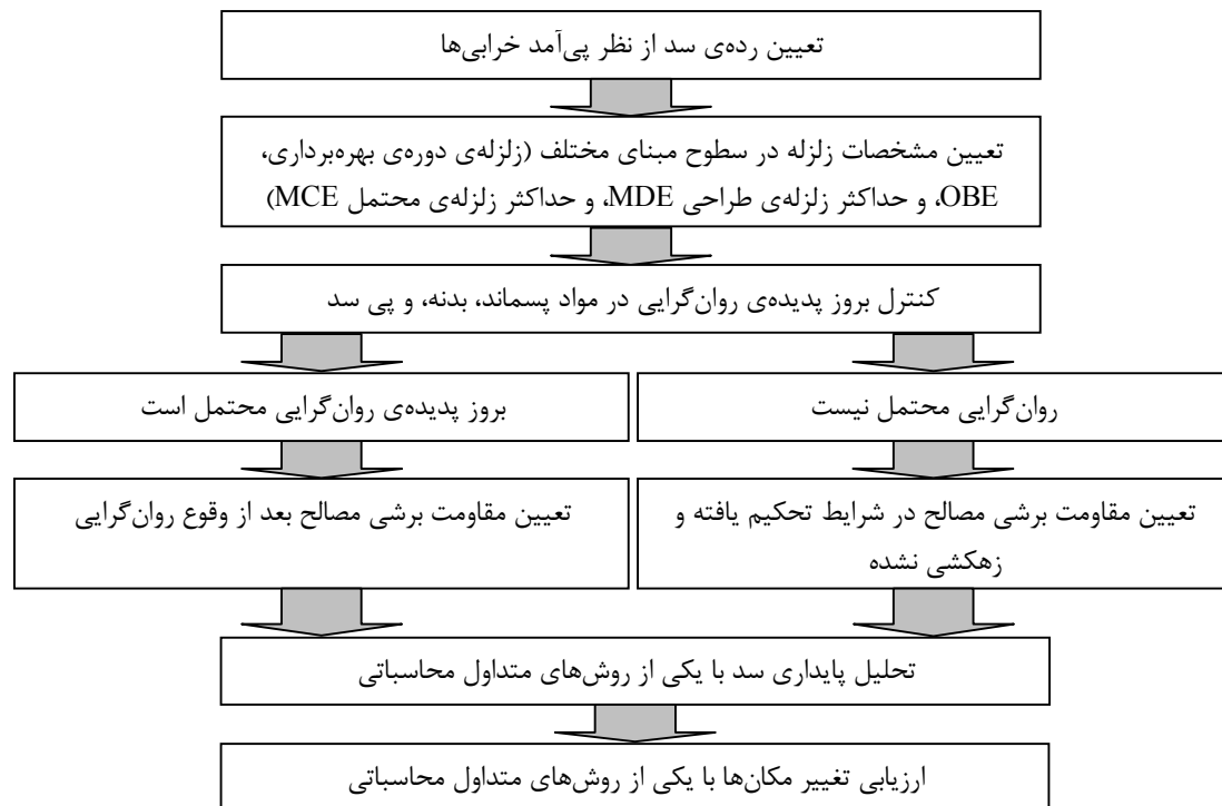
شکل ۶-۱- نمودار روال عمومی تحلیل پایداری سدهای پسماند تحت اثر بارگذاری لرزه‌ای
