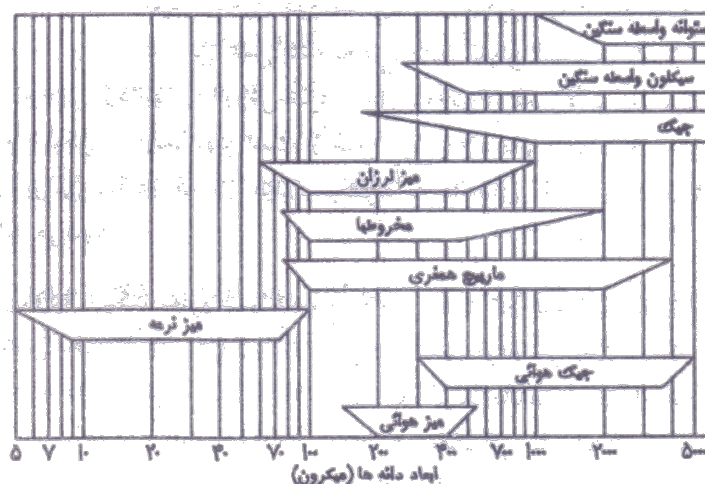
شکل ۱-۱- اندازه مناسب بار ورودی برای دستگاه‌های مختلف جدایش
