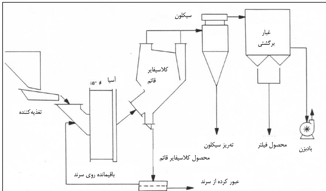
شکل ۱-۱۲- نمای کلی مدار آزمایش شاخص کار آسیای خودشکن مکفرسون
