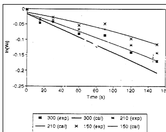
شکل ۲-۴- تغییرات کسر مواد درشت‌تر از چشمه سرن در طی زمان خردایش
