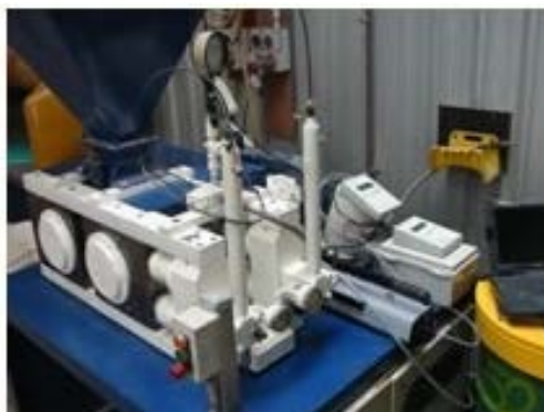
شکل ۱۴-۳- HPGR در مقیاس آزمایشگاهی
