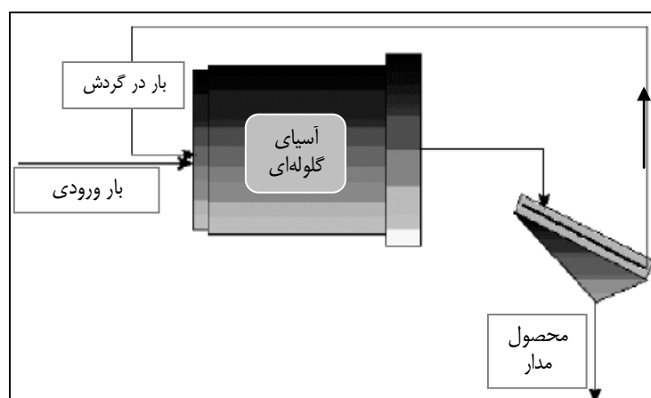
شکل ۱-۱- مدار آزمایش تعیین شاخص کار باند با استفاده از آسیای گلوله‌ای
