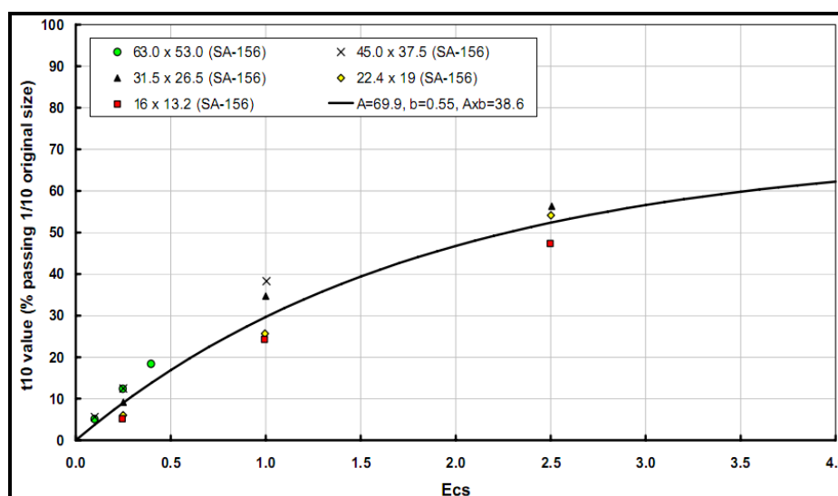
شکل ۴-۱۰- نمودار تغییرات t_{10} بر حسب E_{CS} در آزمایش سقوط وزنه JK
