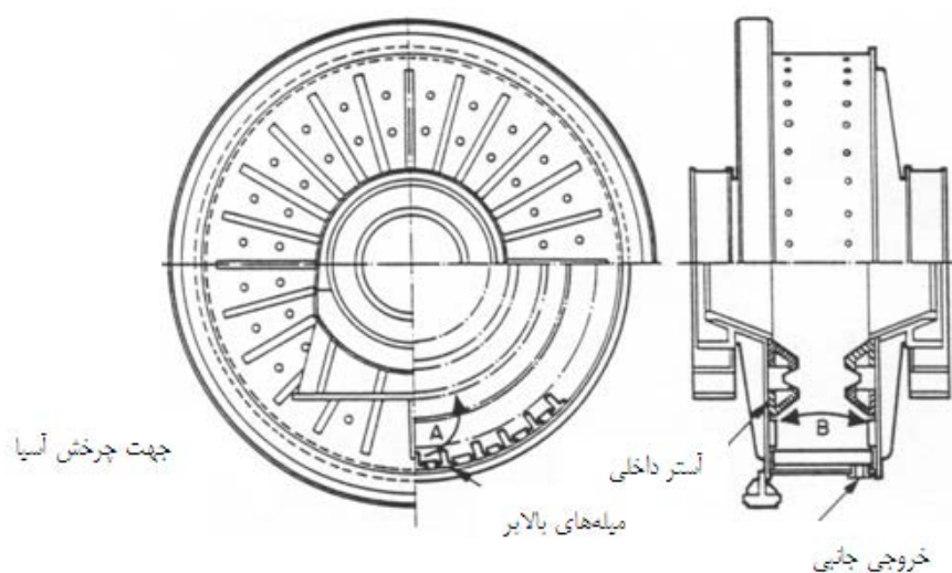
شکل ۱۲-۲- نمای آسیای خودشکن در آزمایش مکفرسون
