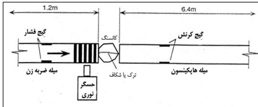
شکل ۹-۱- نمای کلی آزمایش میلۀ فشار هاپکینسون
