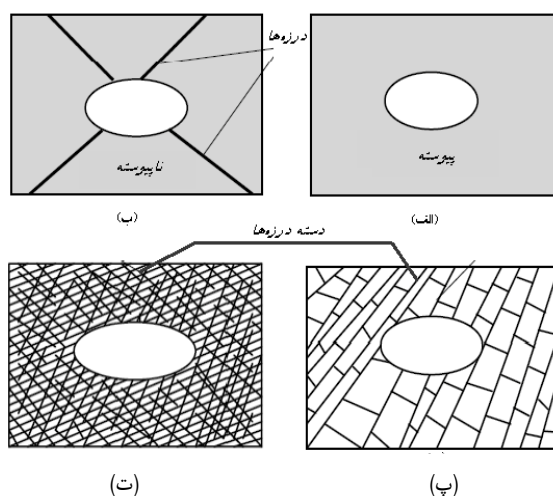
شکل ۶-۲- مناسب بودن روش‌های عددی مختلف برای یک حفیه در توده سنگ: (الف) روش پیوسته، (ب) روش پیوسته با المان‌های درزه و فصل مشترک یا روش اجزای مجزا (ناپیوسته)، (پ) روش ناپیوسته اجزای مجزا و (ت) روش پیوسته با خواص محیط معادل
