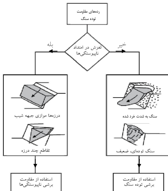
شکل ۵-۱- رابطه بین ساختارهای زمین‌شناسی و رده‌های مقاومتی توده سنگ
