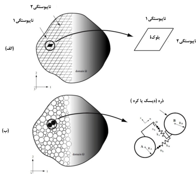
شکل ۲-۵- المان‌بندی در یک دامنه فرضی در روش (الف) اجزای مجزا و (ب) روش ذرات به هم متصل
