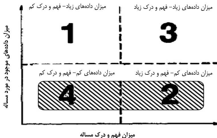
شکل ۱-۱- تقسیم‌بندی مسایل مهندسی بر اساس میزان اطلاعات پیرامون آن‌ها و درک و فهم از مساله
