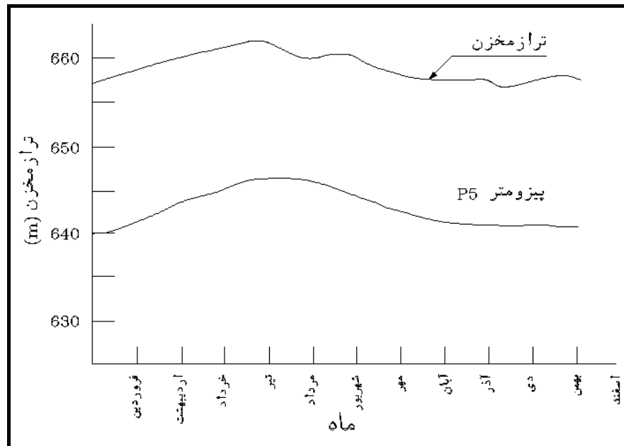
شکل پ. ۵-۴۶- تغییرات تراز پیزومترهای مختلف بر حسب زمان همراه با تغییرات تراز آب مخزن
