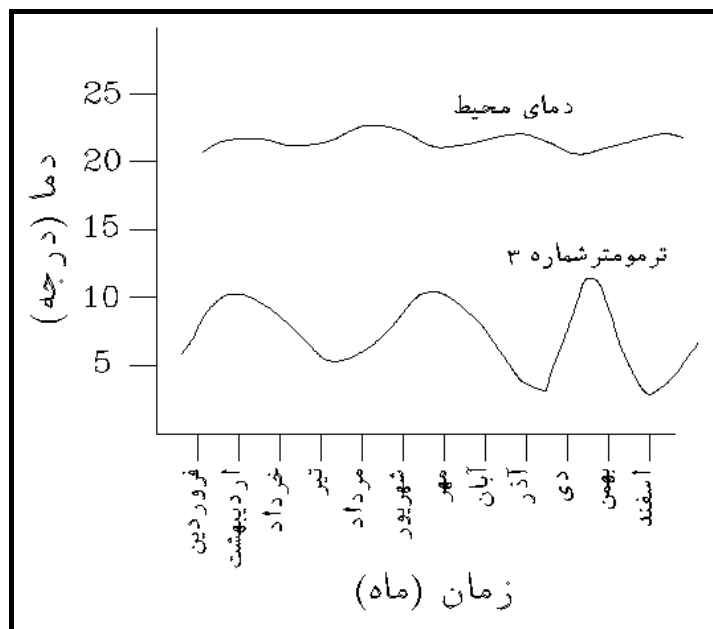
شکل پ. ۵-۴- ترسیم جداگانه تغییرات زمانی دمای هوا و دمای ترمومترهای مدفون در قسمت‌های مختلف سد در رویه بالادست و پایین دست در یک نمودار
