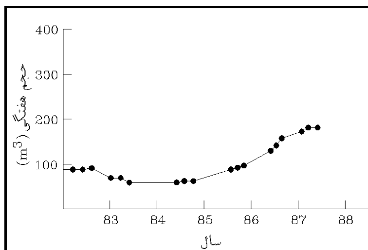
شکل پ.۵-۴-۲-۸-۵-۱- حجم کلی تراوش آب مخزن در طول زمان در تمام یا هر یک از زهکش‌ها
