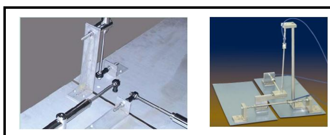
شکل پ. ۵-۲۷- نصب سه بعدی درز سنج
