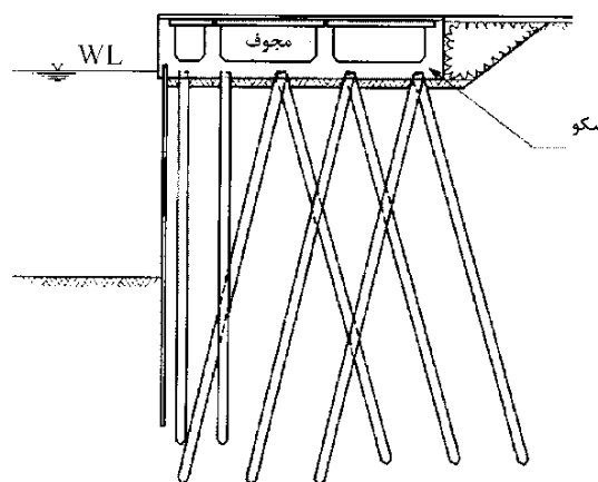
شکل ۸-۲۷- سازه اسکله سپری با سکوی کمکی (عرشه قوطی شکل)
