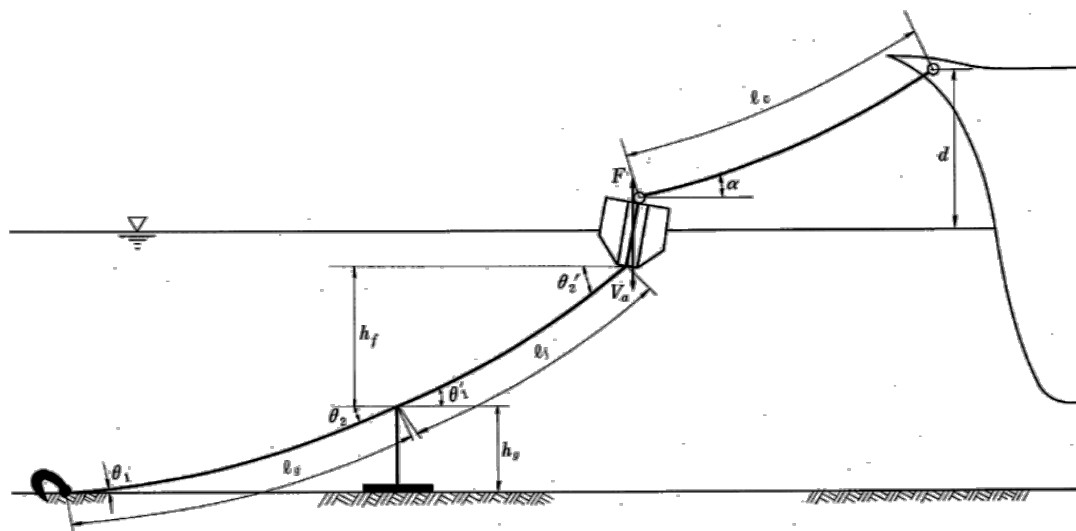
شکل ۸-۸۷- نمایشی از بویه مهاری از نوع ترکیب وزنه و لنگر زنجیری
