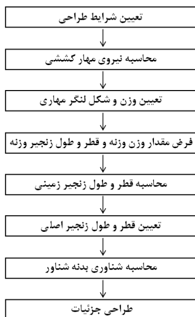
شکل ۸-۸۵- روند طراحی بویه مهاری
