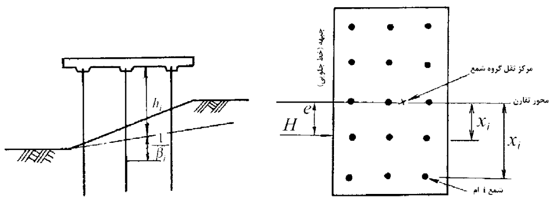
شکل ۸-۶۰- فاصله بین مرکز ثقل گروه شمع و شمع‌های منفرد
