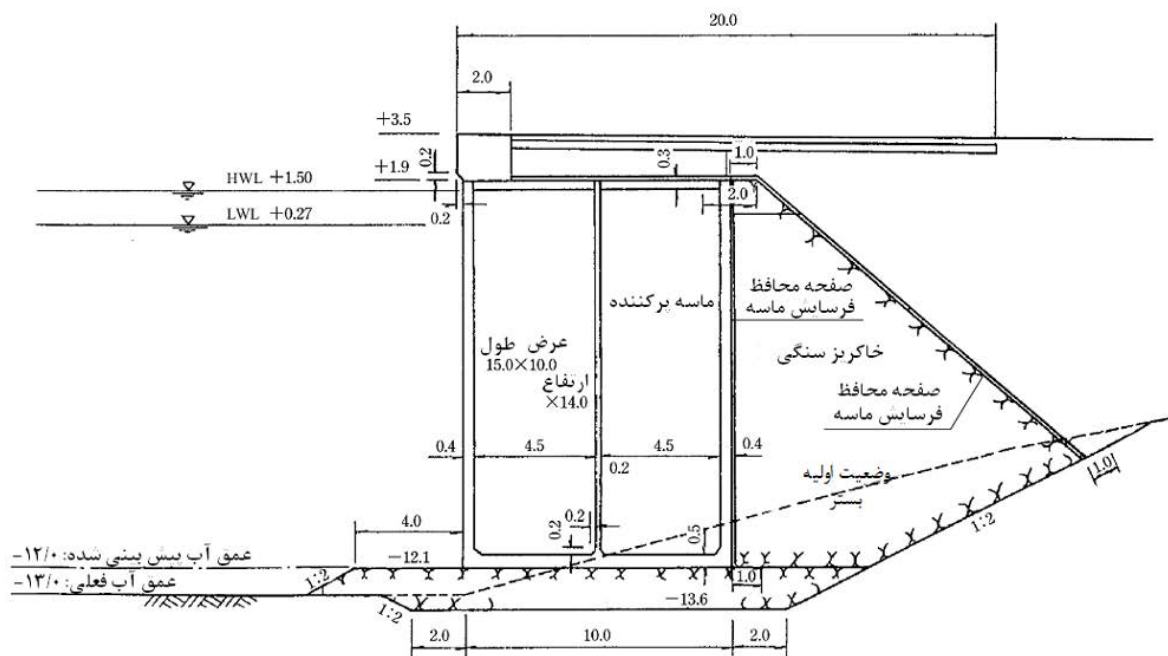
شکل ۸-۳- نمونه‌ای از سطح مقطع یک اسکله دیواری وزنی
