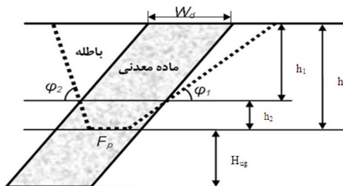
شکل ۴-۲- حالت دوم از وضعیت کانسار و مساله تغییر روش استخراج
