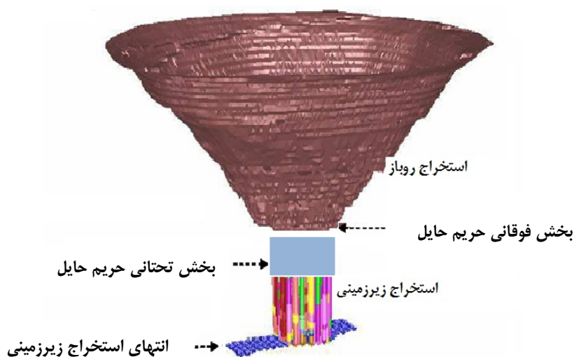
شکل ۱-۱- استخراج ترکیبی روباز و زیرزمینی و مرز تغییر روش استخراج
