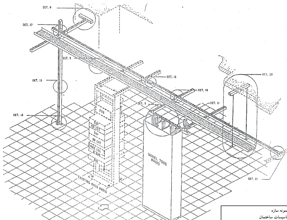
شکل ۵-۲-۱- پایدار سازی تجهیزات رادیو به کف و دیوارها
