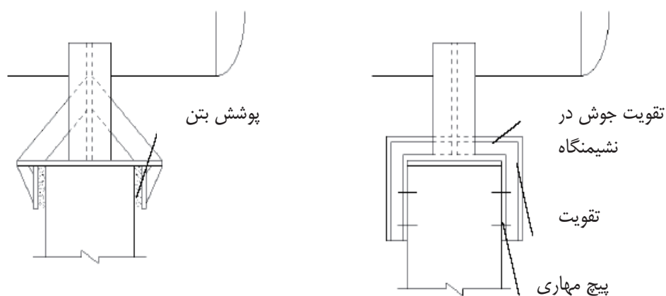
شکل ۵-۱۷ نمونه بهسازی لرزه‌ای پیچ‌های مهری (د)
