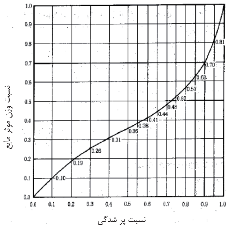
شکل ۲۳-۵ نرخ موثر وزن مایع
