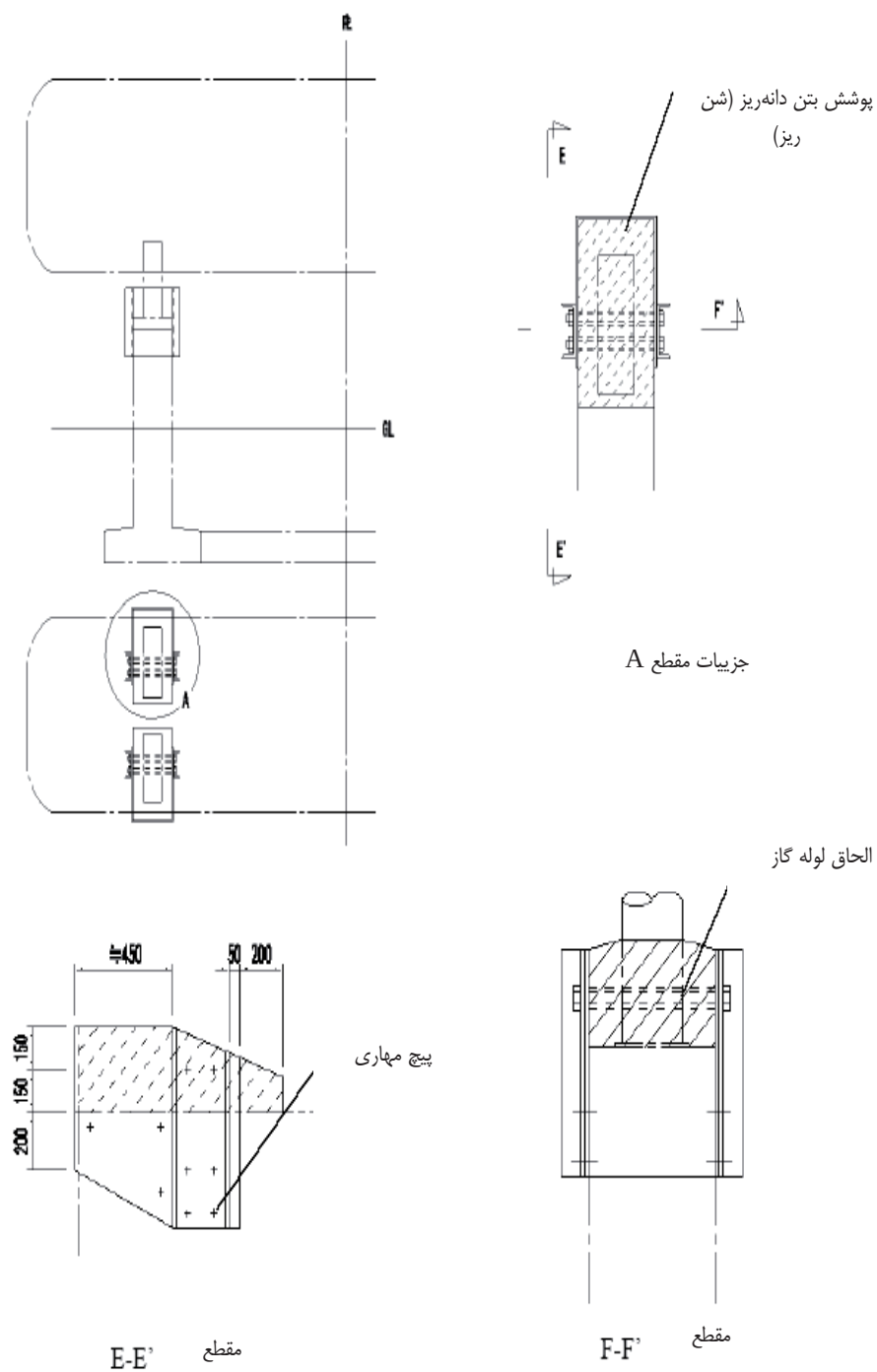
شکل ۵-۱۴ نمونه بهسازی لرزه‌ای پیچ‌های مهری (الف)
