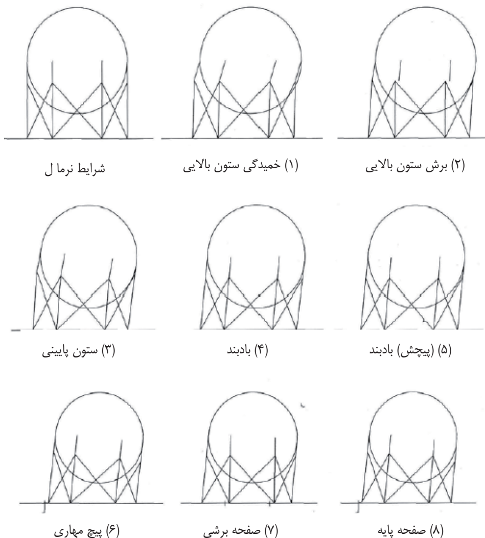
شکل ۵-۲۷ انواع آسیب به مخازن کروی
