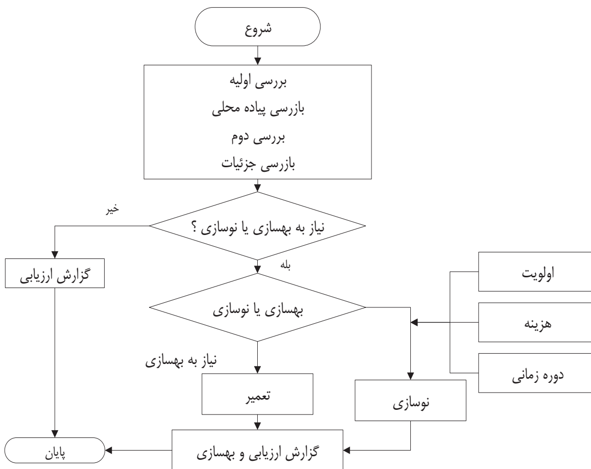
شکل ۳-۷ روند ارزیابی لرزه‌ای خط لوله روزمینی و پل لوله
