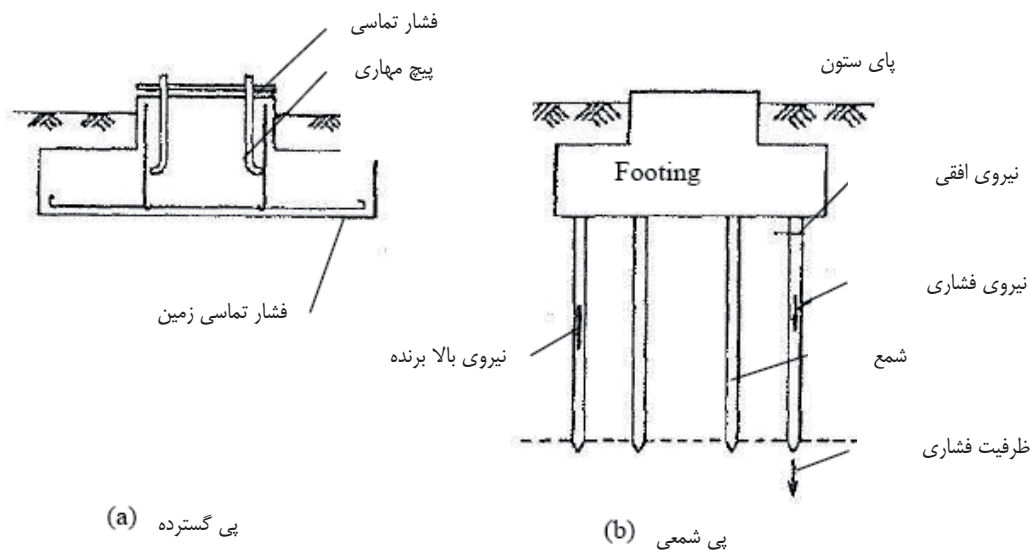
شکل ۵-۳۹ حالت‌های آسیب‌دیدگی پی
