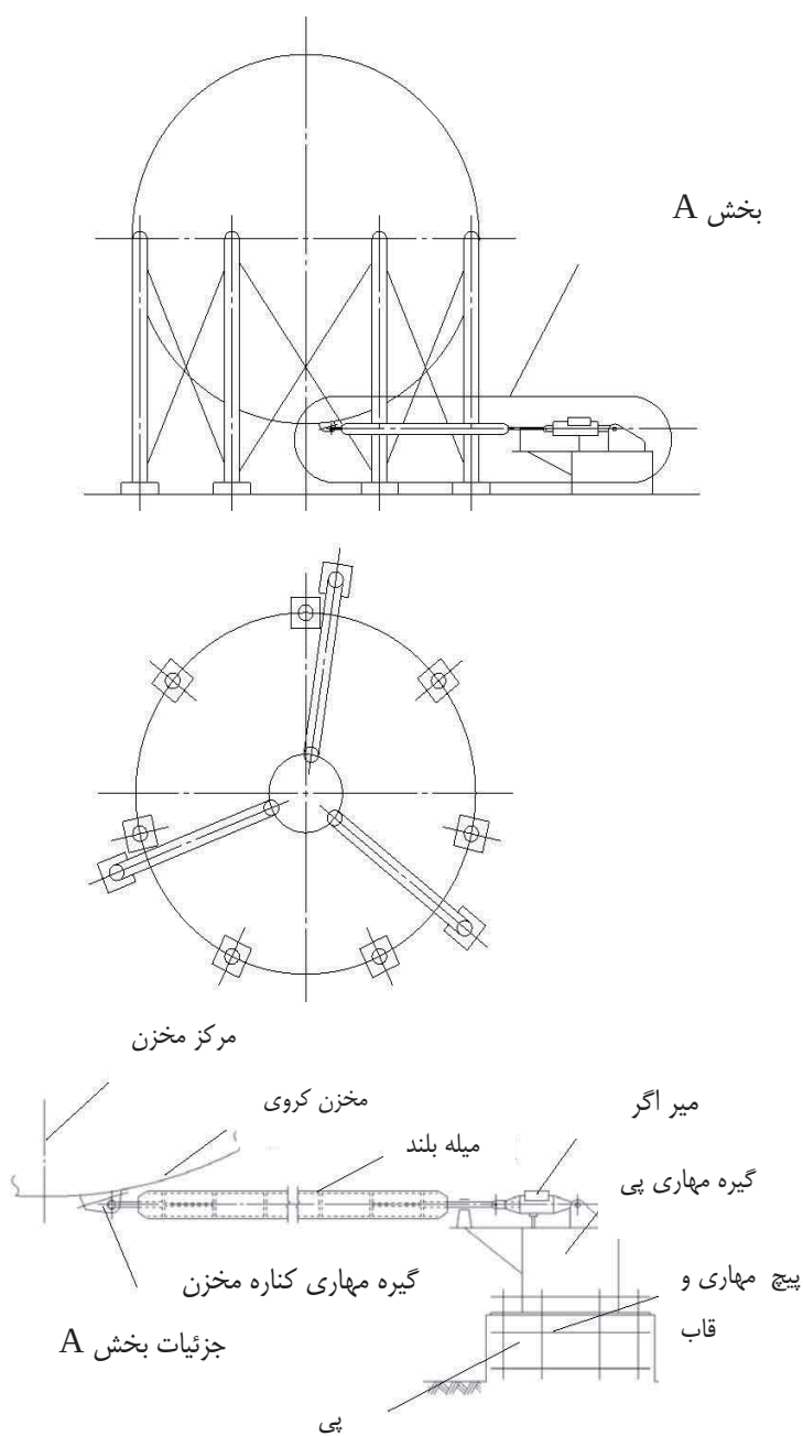
شکل ۵-۳۵ کنترل ارتعاش با استفاده از میراگر (از نوع میله بلند)
