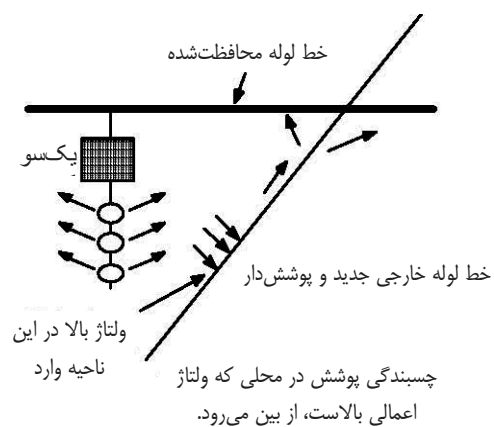
شکل ۷-۸ تداخل ولتاژ
