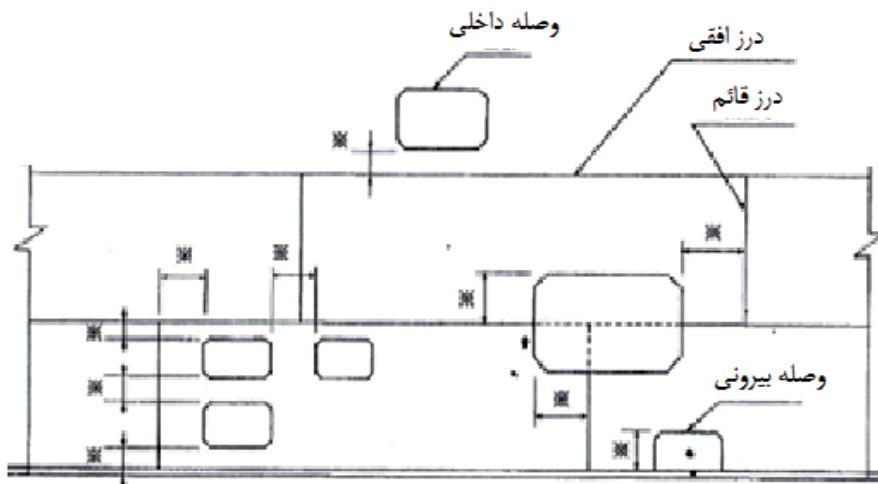
حداقل فواصل علامت‌گذاری شده ۵۰ میلی‌متر یا ۸t است که t ضخامت پوسته مخزن می‌باشد.
