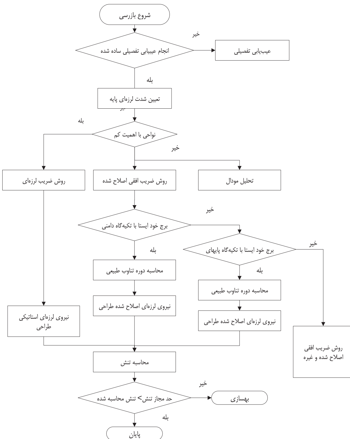
شکل ۵-۲۵ روند نمای روند طرح بهسازی برای ارتقاء مقاومت لرزه‌ای
