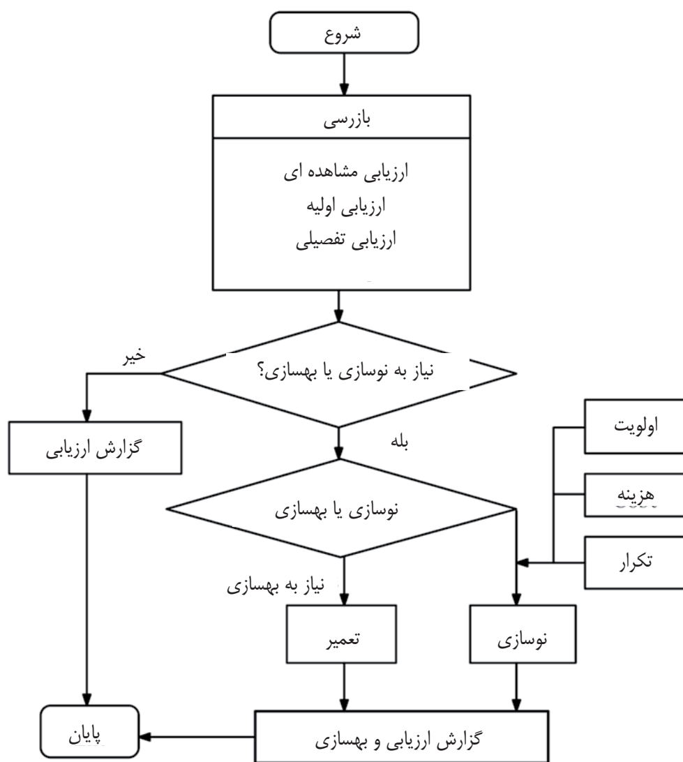
شکل ۱۰-۳ روند نمای ارزیابی و بهسازی لوله‌ای کالورت
