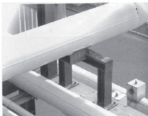
شکل ۵-۲ جداشدگی لوله از محل نشیمن‌گاه در اثر شتاب پاسخ
