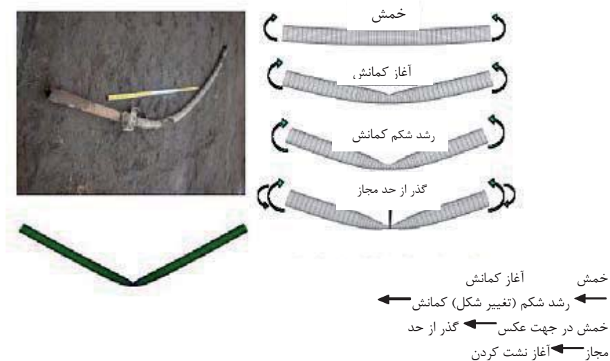
شکل ۸-۲ لوله تغییر شکل یافته بر اثر زمین لرزه
