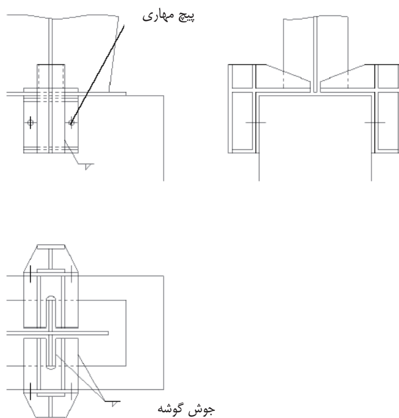
شکل ۵-۱۷ نمونه بهسازی لرزه‌ای پیچ‌های مهری (د)
