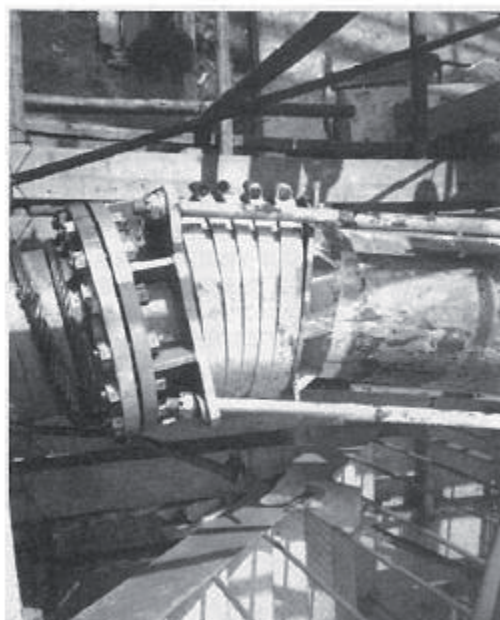
شکل ۳-۵ از دست رفتن عملکرد مفصل لوله انعطاف‌پذیر
