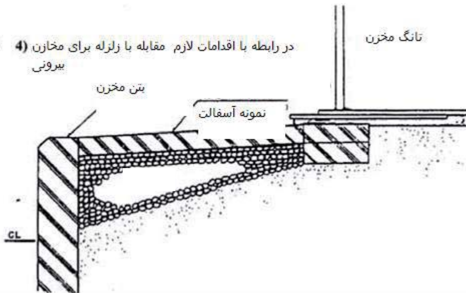
شکل ۶-۲۱ روش تقویت پی مخازن
