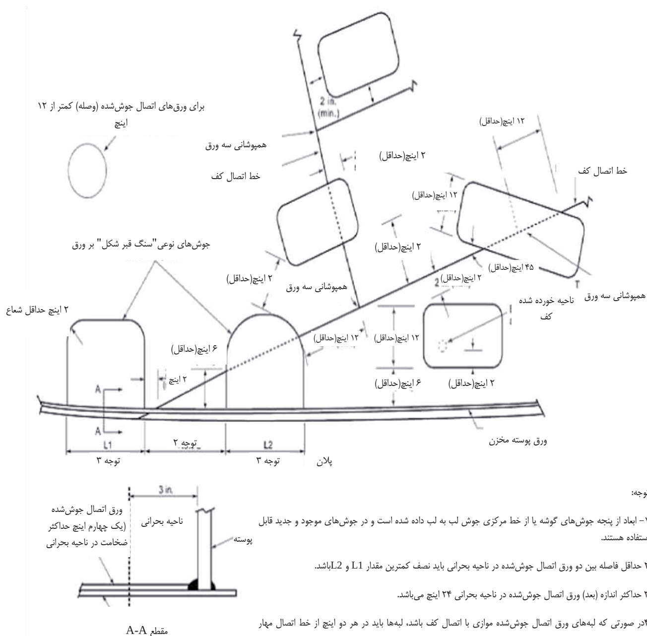
شکل ۶-۱۴ ورق‌های اتصال جوشی در کف مخازن
