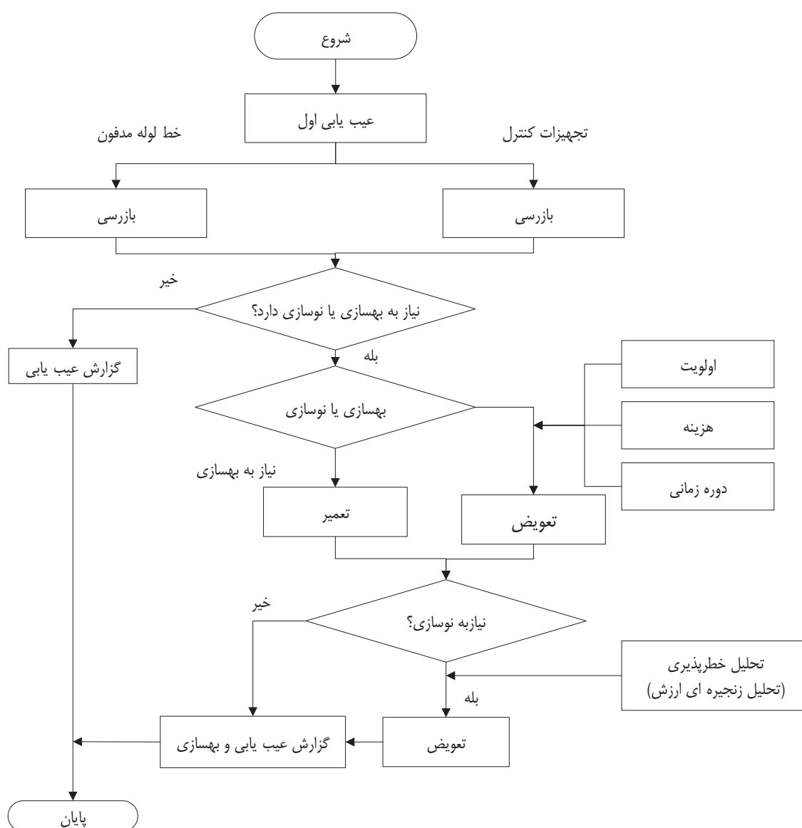
شکل ۸-۴ روند ارزیابی لوله‌ای خط لوله مدفون و تأسیسات کنترل آن
