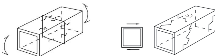
ترک‌های بخش اتصال ناشی از تغییر شکل خمشی
