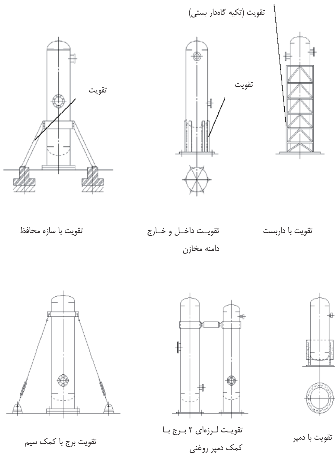
شکل ۵-۲۶ بهسازی لرزه‌ای برج
