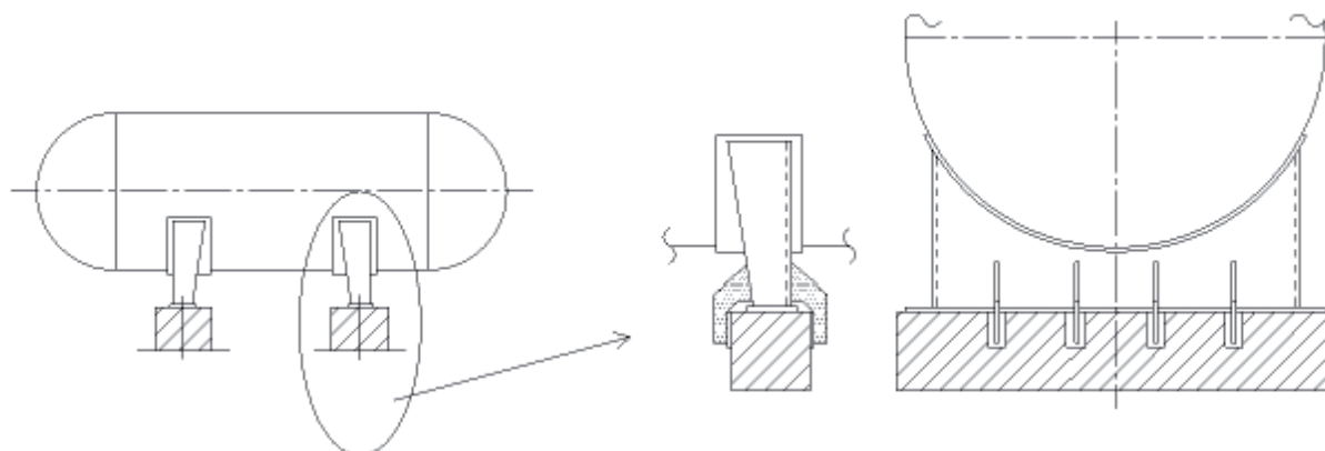
شکل ۵-۱۹ نمونه بهسازی لرزه‌ای پیچ‌های مهار (ز)
