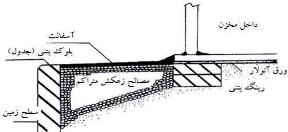
شکل ۶-۲۳ روش حفاظت تصفیه آب باران با استفاده از آب‌بند
