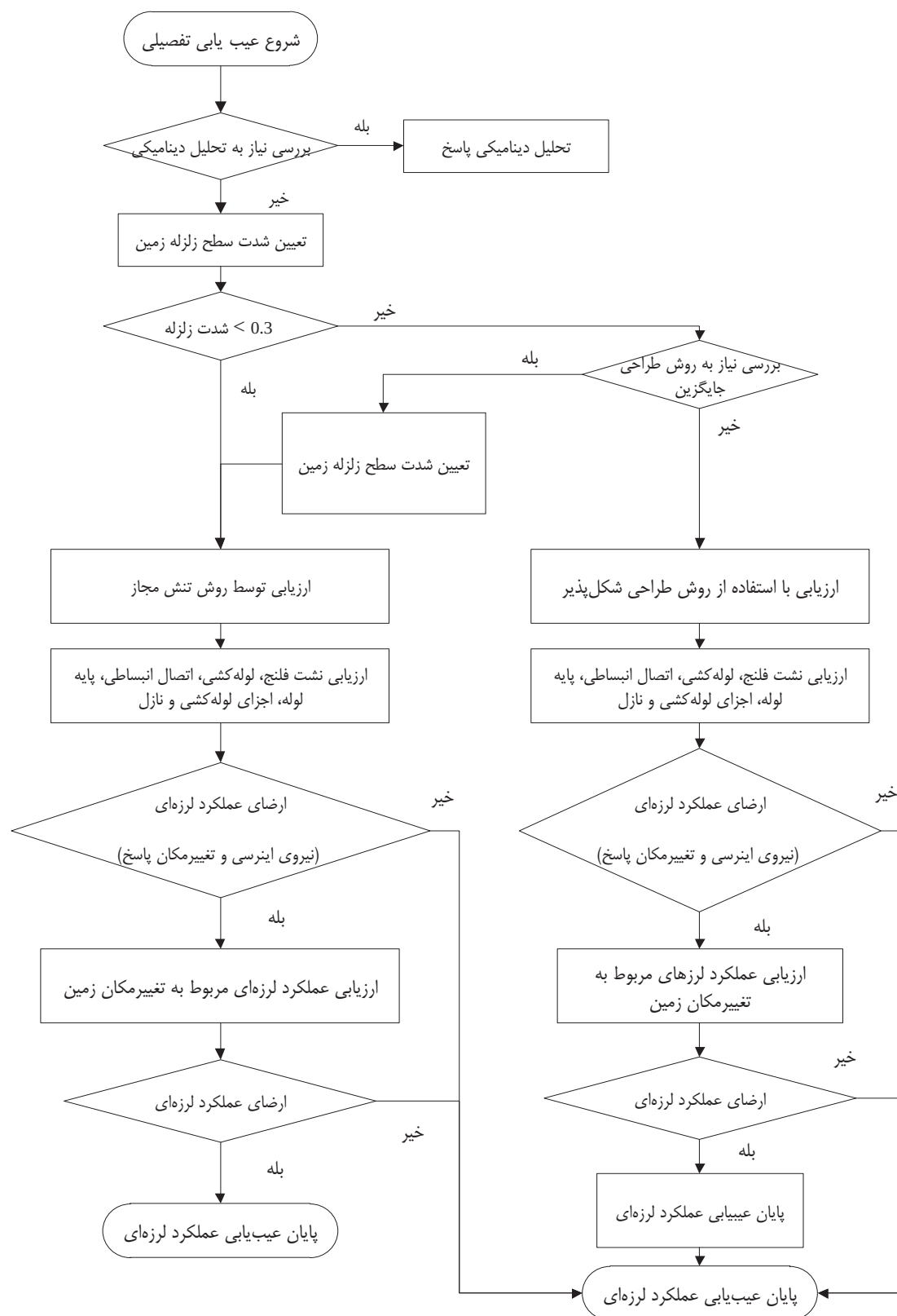
شکل ۷-۵ روند نمای ارزیابی تفصیلی
