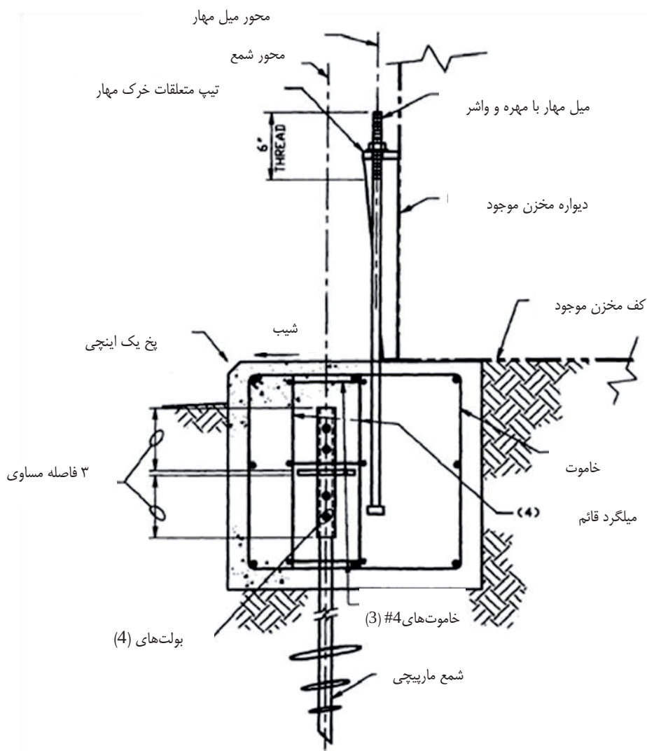
شکل ۶-۲۲ شمع‌های مارپیچ بکار رفته با پی دیواره حلقوی
