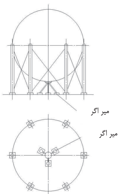
شکل ۳۶-۵ کنترل ارتعاش با استفاده از میراگر با مواد ویسکو-الاستیک
