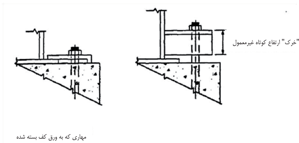
شکل ۶-۲۵ جزئیات ضعیف مهاربندی
