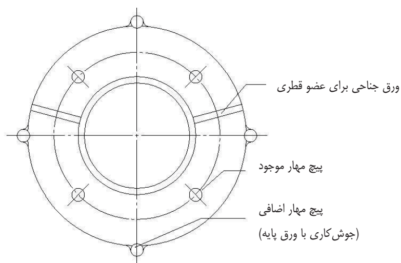
شکل ۵-۳۲ اضافه کردن زبانه مهار
