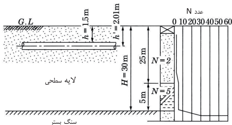
شکل ۲-۸-۱۴ - پروفیل خاک
