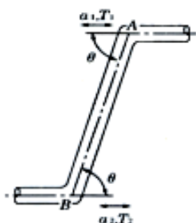
(ب) حالتی که تنش خمشی در پایه‌های پل زیاد است
