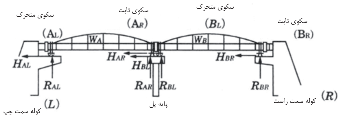
شکل ۷-۲۲ نمونه نیروی اینرسی وارد بر پل (دو دهانه (A و B)، دو کوله (L و B) و یک پایه (در وسط))
