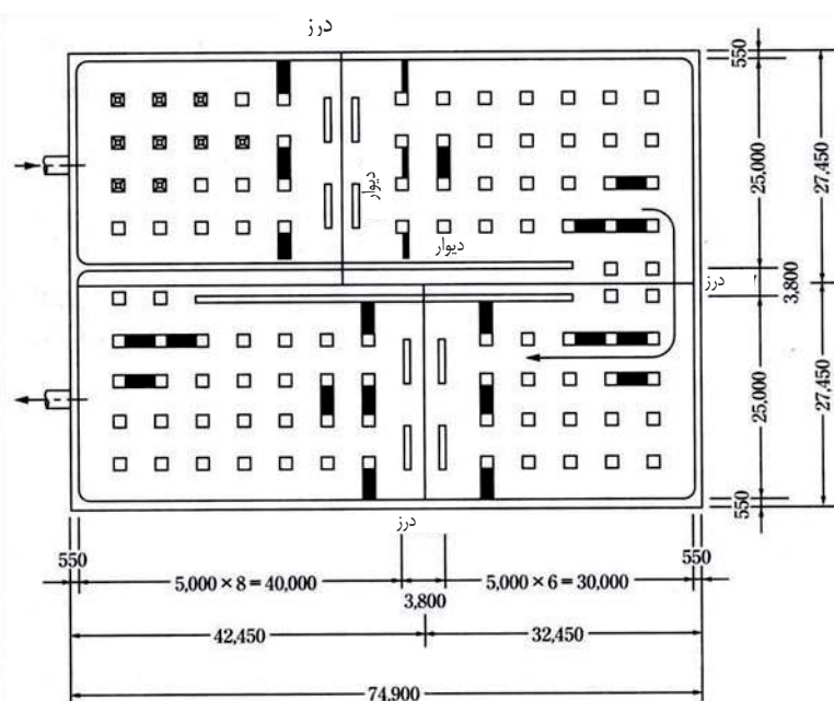
شکل ۵-۴ نمونه‌ای از یک حوضچه با دیوارهای برشی داخلی
