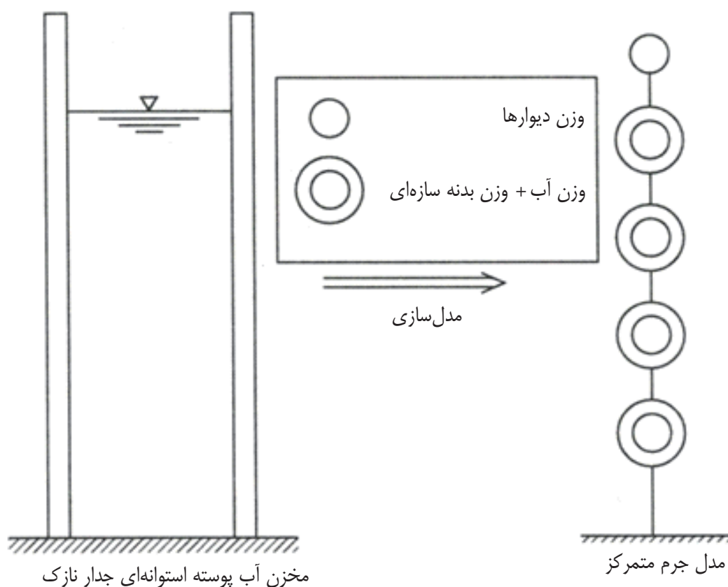
شکل ۶-۱ مدل تحلیل دینامیکی
