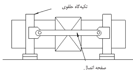
نوع ۳ اتصال دو طرفه روسازه به هم
