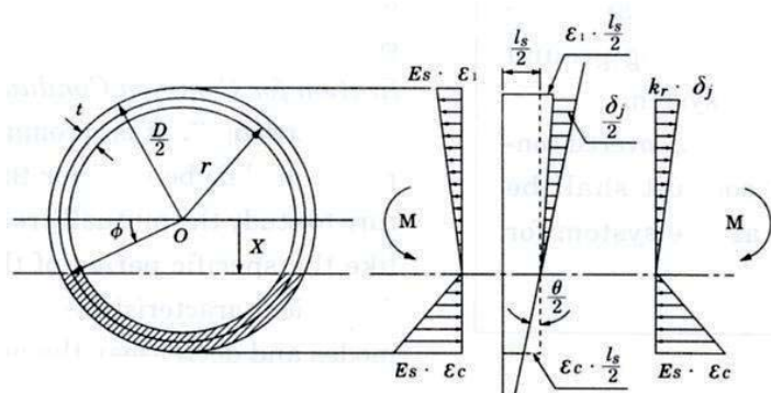
شکل ۷-۲۱- مرحله اول- تنش مرکب و تغییر مکان حلقه اتصال (هنگامی که نیروی کنشی در مرحله ارتجاعی است)
