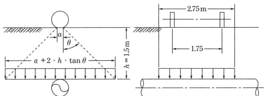
شکل ۸-۱۰- توزیع بار وسیله نقلیه بر لوله
