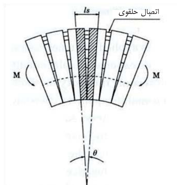
شکل ۷-۲۰ مکانیزم تغییر شکل قطعه اتصال تحت ممان خمشی
