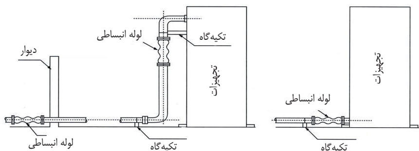
شکل ۴-۵ لوله‌های اطراف مخازن و تجهیزات
