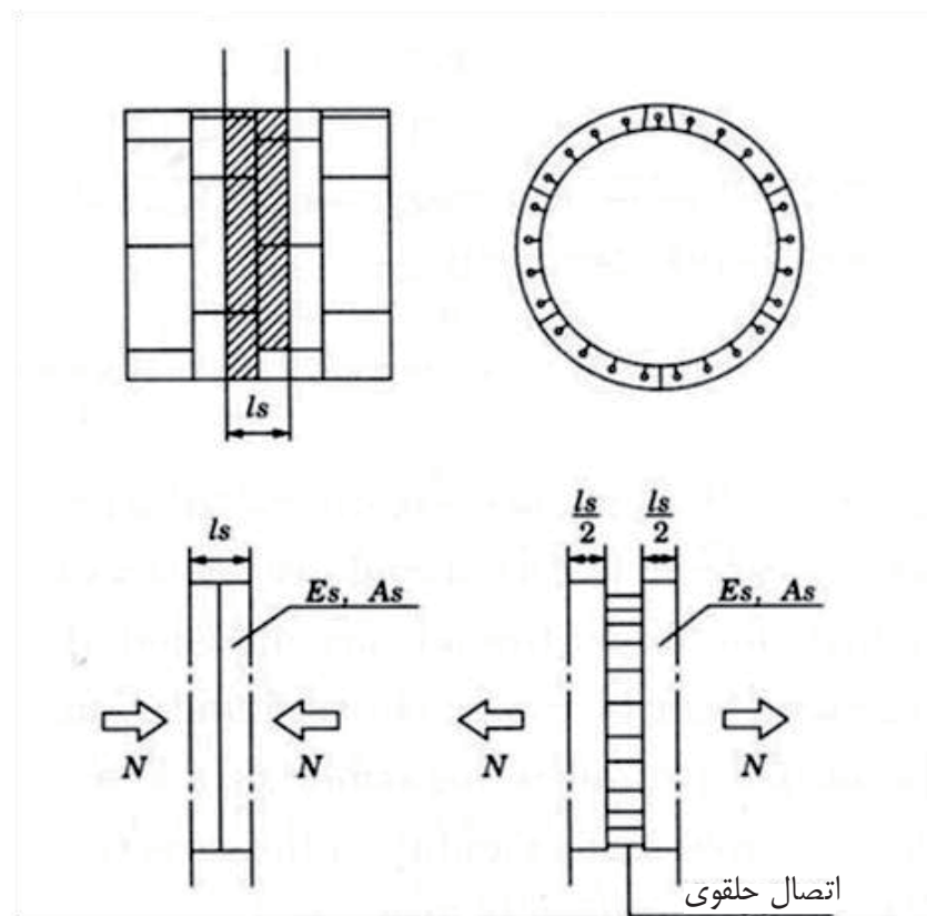
شکل ۷-۱۹ ارزیابی سختی محوری معادل
