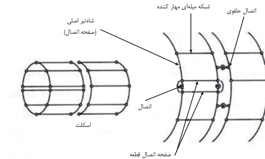
شکل ۷-۱۶ مدل ساخت سپر قاب‌بندی شده فاصله‌دار تونل سپری
