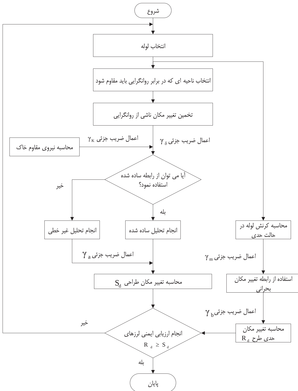
شکل ۷-۹ نحوه اعمال ضرایب جزئی ایمنی
