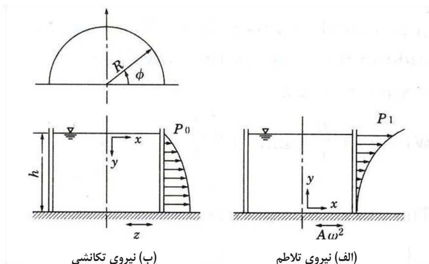
شکل ۳-۶ مدل فشار آب Housner
