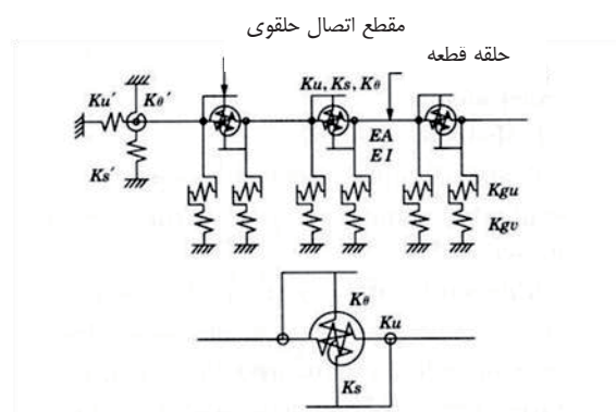
شکل ۷-۱۸ مدل ساخت استوانه‌ای طولی تونل سپری
