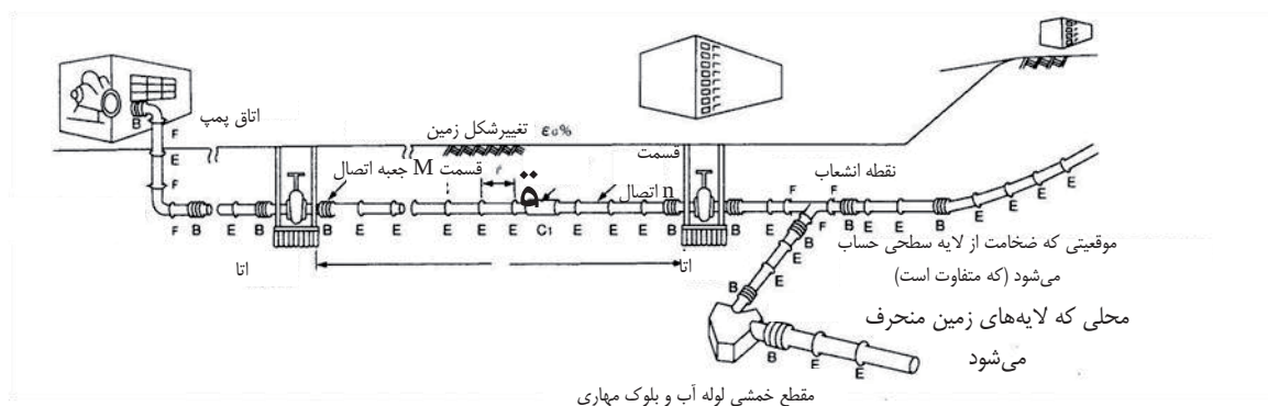
شکل ۷-۵ طرح تصویری خط لوله گسسته
