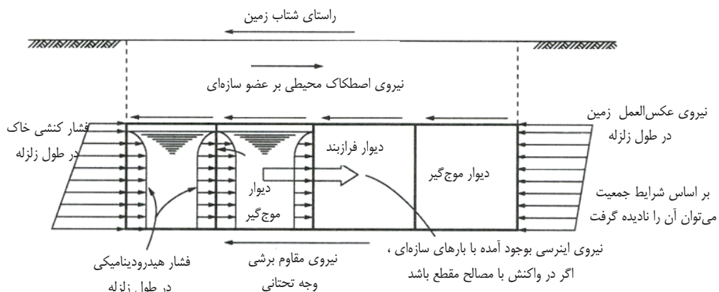
شکل ۵-۱ نمونه بار زلزله (یک سمت مخزن پر/طرف دیگر مخزن خالی)
