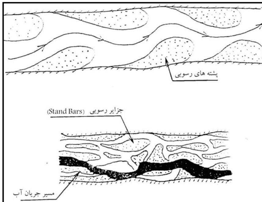
شکل ۲-۱۱- نمونه‌هایی از تشکیل جزایر و بشته‌های رسوبی در بستر رودخانه‌ها [۱۳]
