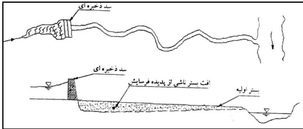
شکل ۲-۶- پدیده کف‌کنی مستمر در پایین دست سد مخزنی [۱۳]
