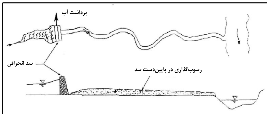
شکل ۲-۷- نحوه رسوب‌گذاری در پایین دست سد انحرافی [۱۳]
