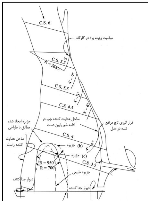
شکل ۵-۲۷- جزئیات طراحی کناره‌های هدایت کننده جریان و جزیره مرکزی آن در مدل اصلاح شده سد انحرافی کورتی در پاکستان [۳۷]
