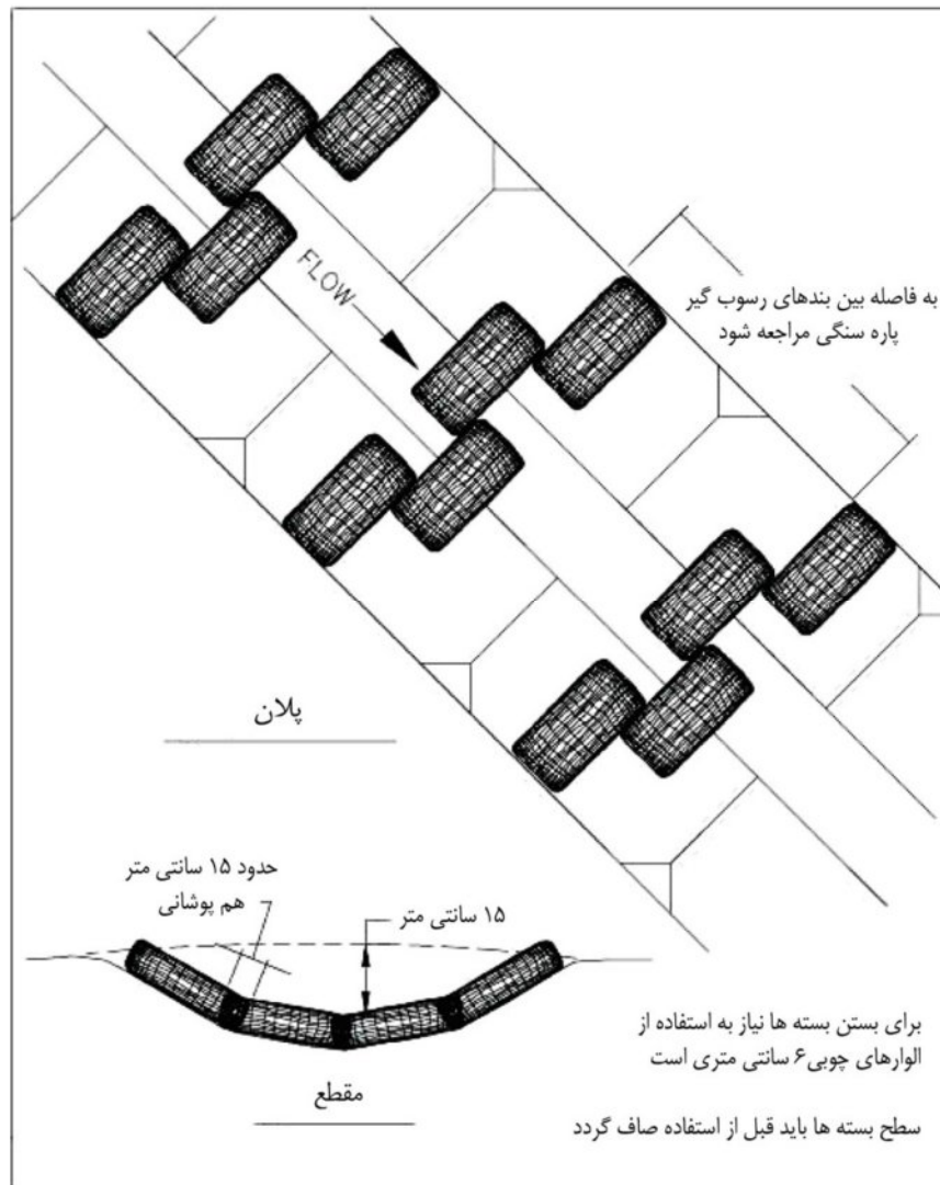
شکل ۵-۱۲- نمایشی از سد رسوب‌گیر با بسته‌های پر شده در آبراهه
