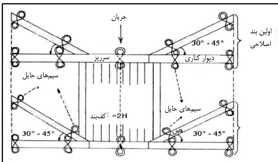
شکل ۵-۹- تصویر اولین سد اصلاحی الواری همراه با پیش بند
